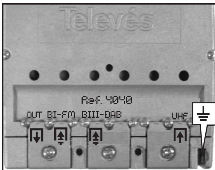
Označení vstupů, nastavení zesílení, zemnění
